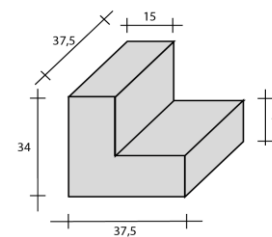
Rinnenbordstein 37,5/34/37,5
