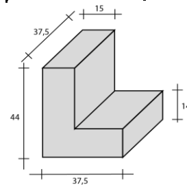
Rinnenbordstein 37,5/44/37,5
